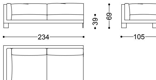
El.Terminale 4 posti con 1 bracc. sx/dx cm.254 234x105x69 cm - 92.1x41.3x27.2"
