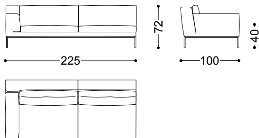
Elemento terminale 3,5 posti sx/dx cm.225 225x100x72 cm - 88.6x39.4x28.3"
